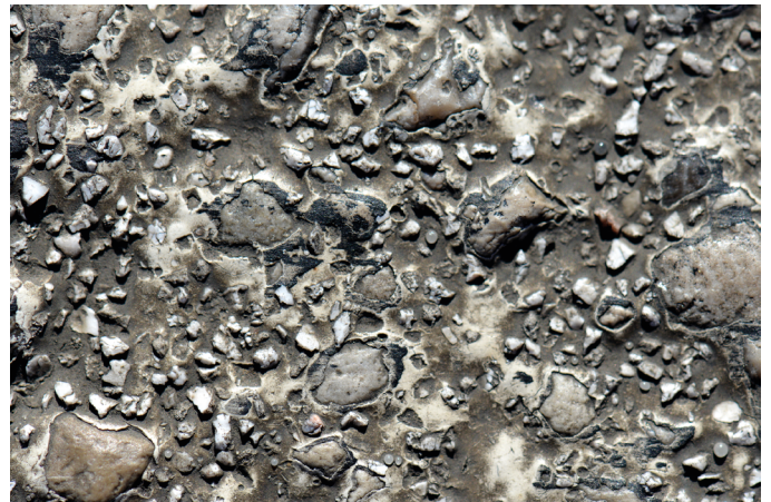
Fig. 5. Close-up image (magnification 3x) of the most used area of sample MG after 10 months Rys. 5. Powiększenie (3x) najbardziej zużytego obszaru oznakowania w obrębie próbki MG po 10 miesiącach
