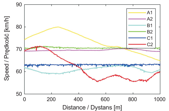
Fig. 2. Vehicle speeds on the test sections Rys. 2. Prędkości pojazdu na odcinkach testowych
