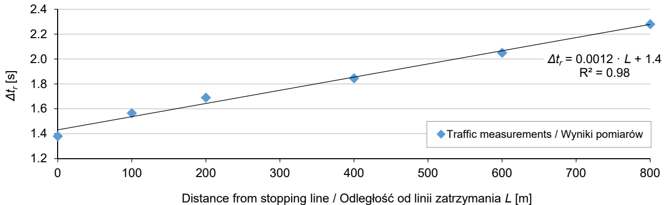
Fig. 5. Average time intervals between the moments in which successive vehicles in the queue start moving Rys. 5. Średnie odstępy czasu pomiędzy ruszaniem kolejnych pojazdów w kolejce
