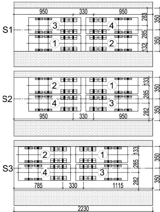
Fig. 3. Location of vehicles in subsequent load schemes Rys. 3. Ustawienie pojazdów w poszczególnych schematach obciążenia
