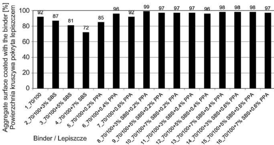
Fig. 4. Results of the visual assessment of binder-aggregate adhesion after the boiling test Rys. 4. Zestawienie wyników oceny wizualnej adhezji lepiszcza do kruszywa po teście gotowania
