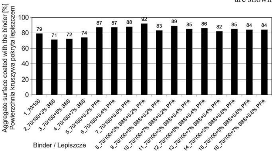
Fig. 5. Results of the computer assessment of binder-aggregate adhesion after the boiling test Rys. 5. Zestawienie wyników oceny komputerowej adhezji lepiszcza do kruszywa po teście gotowania
