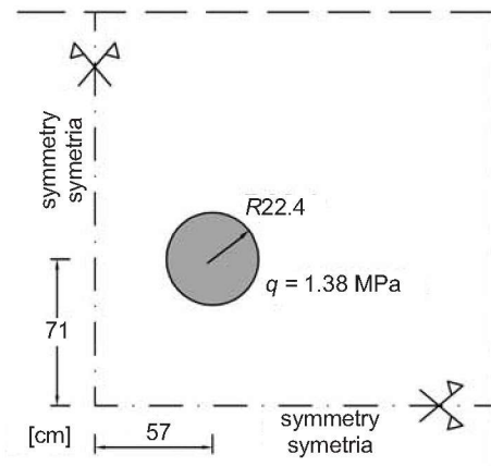
Fig. 3. Loading scheme for flexible pavement structure under the B767-200 aircraft main gear Rys. 3. Obciążenie podatnej nawierzchni lotniskowej golenią główną samolotu B767-200
