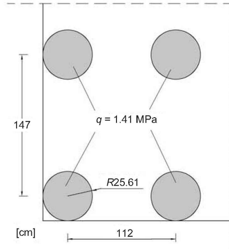
Fig. 1. Loading scheme for concrete plate under the B747-400 aircraft main gear Rys. 1. Schemat obciążenia płyty betonowej golenią główną samolotu B747-400
