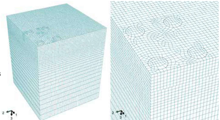
Fig. 6. FEM mesh Rys. 6. Siatka MES
