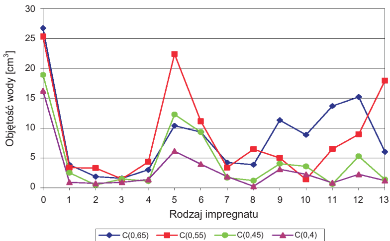
Rys. 6. Wyniki badania wnikania wody Fig. 6. Results of water penetration
